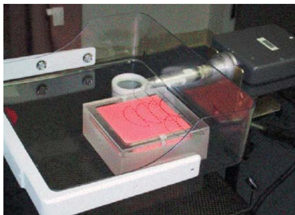
Figura 1. Colocación del maniquí de acreditación y cámara de ionización para realizar las mediciones de la dosis glandular promedio.
