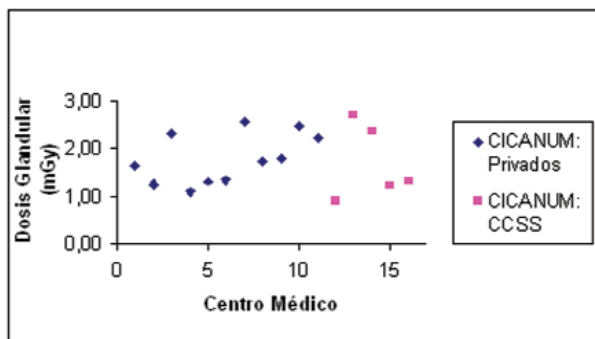
Figura 3. Valor del dosis glandular promedio (mGy) para centros privados y de la CCSS evaluados por el personal del CICANUM-UCR. Valor máximo recomendado internacionalmente 3 mGy.
